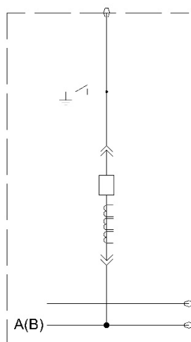
Ячейка КРУ фидера КС
