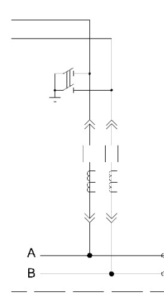
Ячейка КРУ двухфазного СВ
