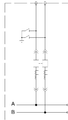
Ячейка КРУ двухфазного фидера ТСН
