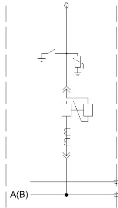
Ячейка КРУ фидера УК
