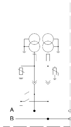
Ячейка КРУ двухфазного ТН
