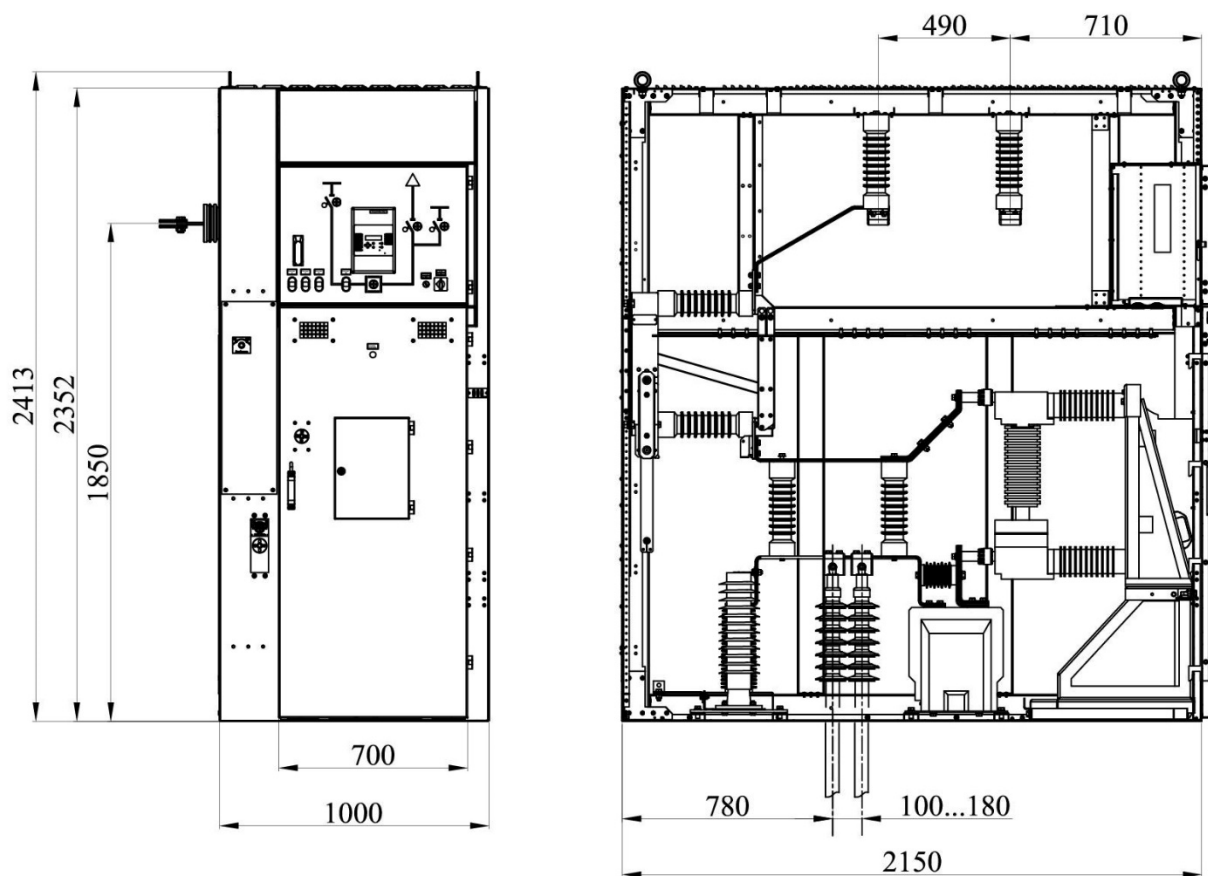
Ячейка однополюсного выключателя серии KR-27,5STS
